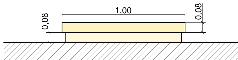
DETTAGLIO TIPO (prospetto) del coperchio tombale
