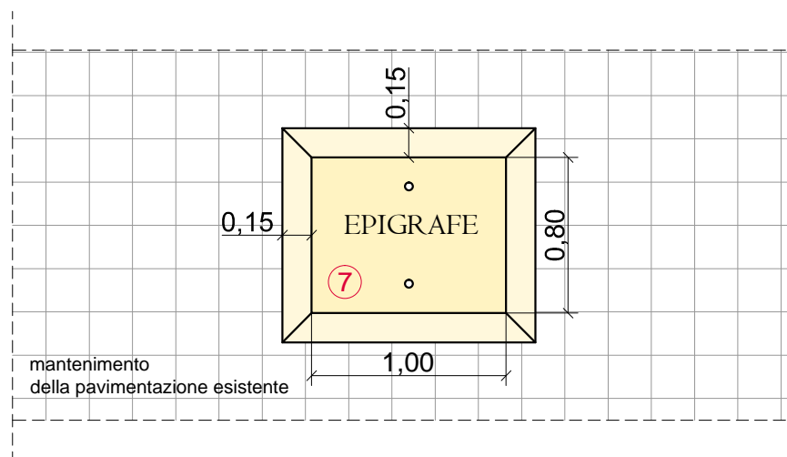
PIANTA TIPO dettaglio del coperchio
