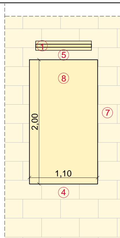
PIANTA - coperchio 110 cm
